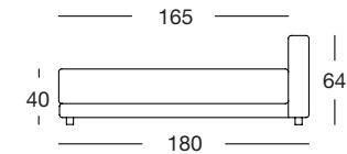
ARB-PSZ 142/ASE-PSZ 142
